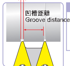
寸法 Dimension(mm)
